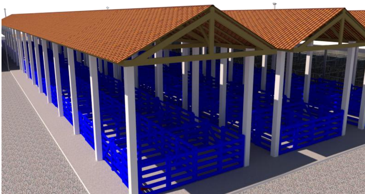
Figura 02 – Layout da Baía 01 da Capritânia 2026
