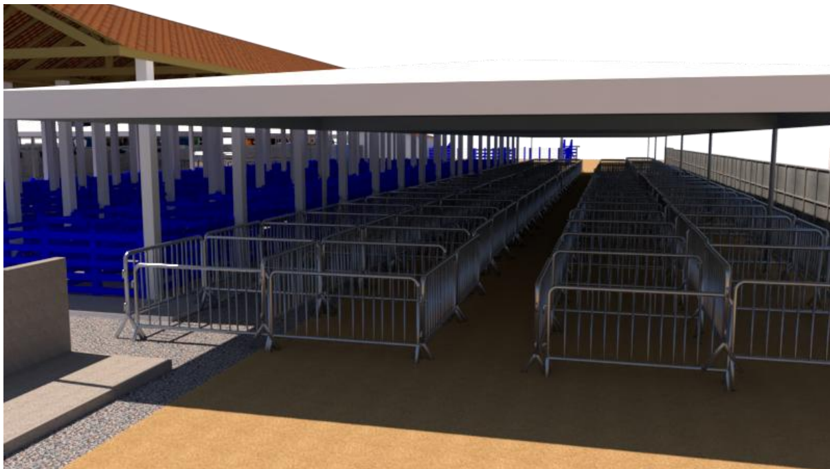
Figura 03 – Layout da Baía 02 da Capritânia 2026
